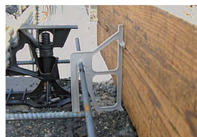
▲木製型枠施工写真
