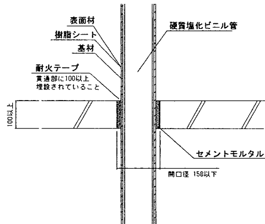
側断面図
