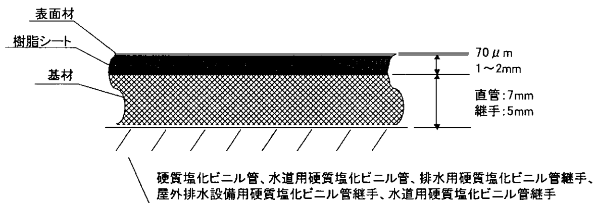
図-1 耐火防音カバー付管及び耐火防音カバー付管継手の構造
