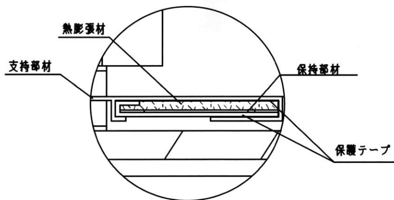
B 部詳細
