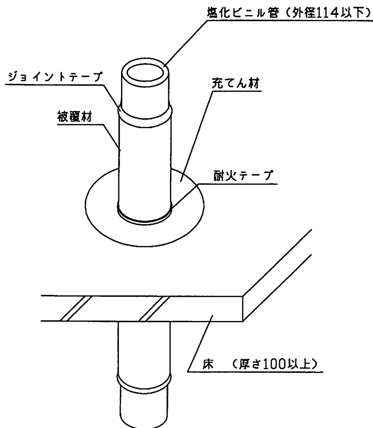
部分被覆の場合
