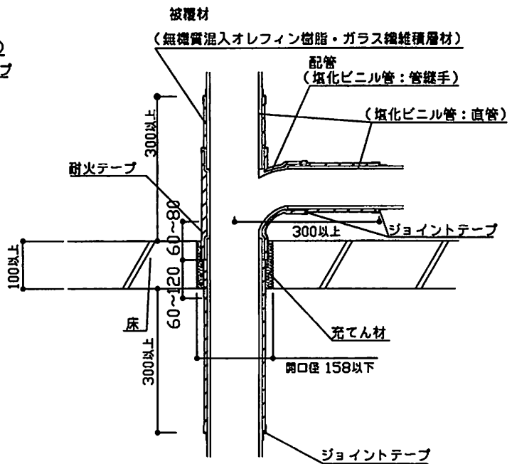
断面図 (部分被覆の場合)
