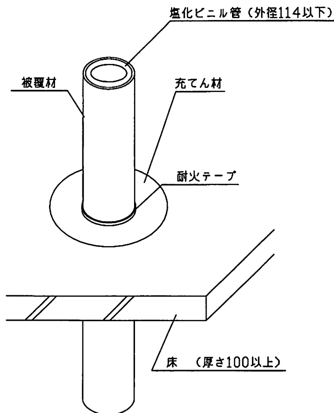
全管被覆の場合
