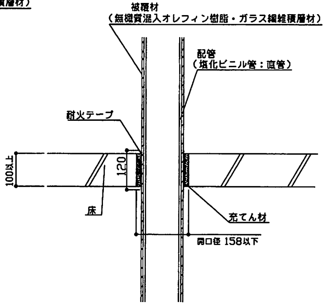
断面図 (全管被覆の場合)
