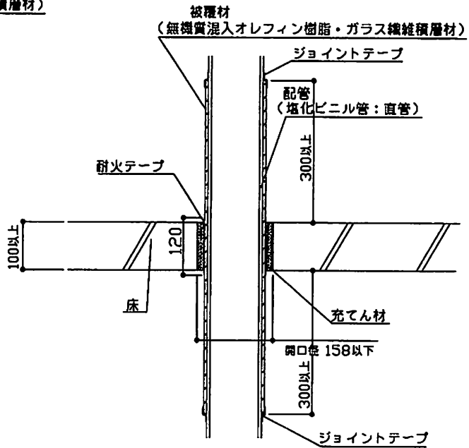
断面図 (部分被覆の場合)
