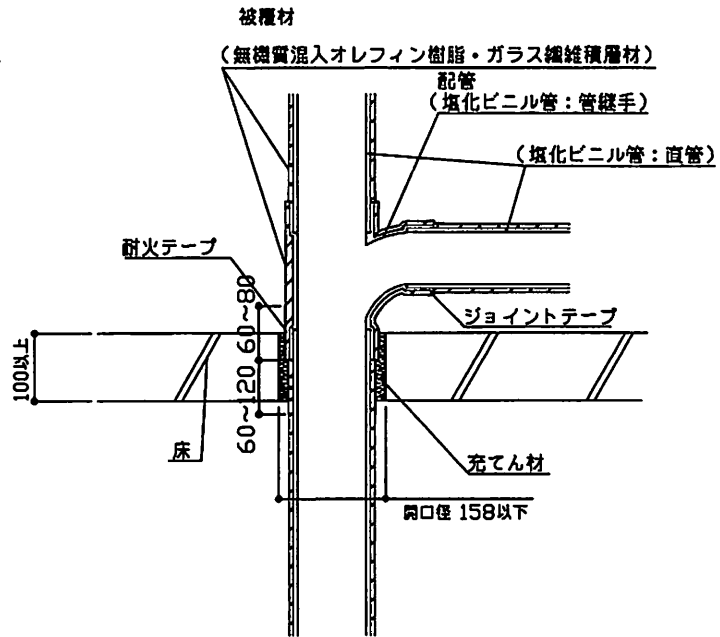
断面図 (全管被覆の場合)
